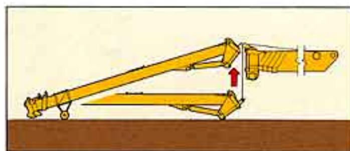
●スーパーラフィングジブの取付
