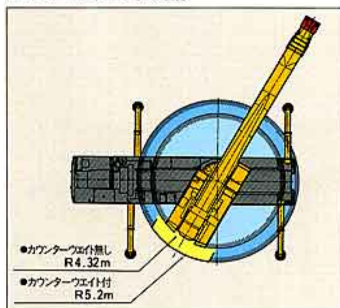
●スーパーラフィングジブの取付
