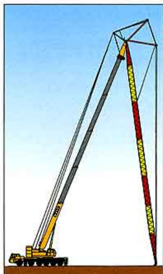
●ヘビーリフトジブの立組
